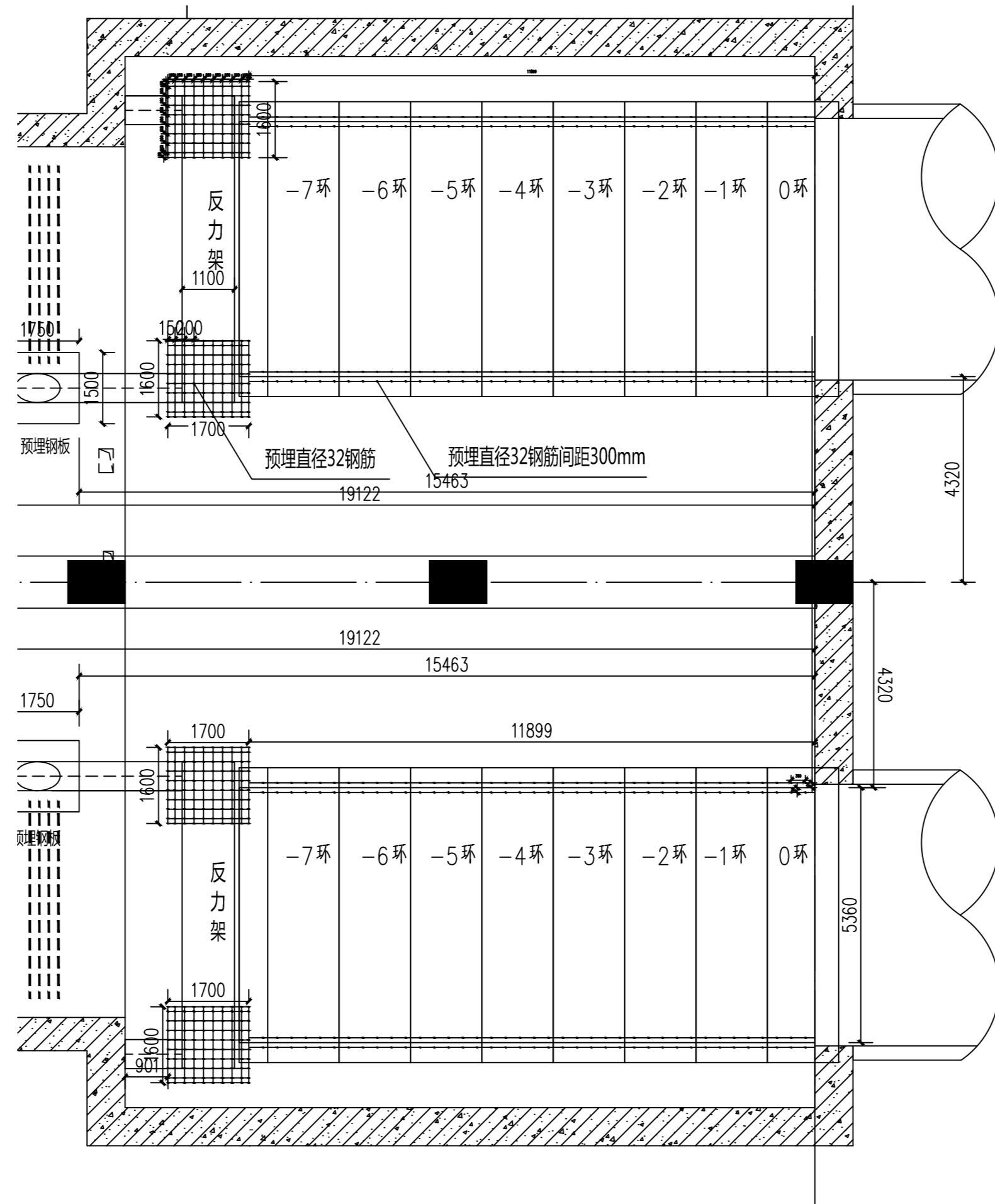
内蒙古体育场馆站区间盾构始发洞衬砌性平面图
