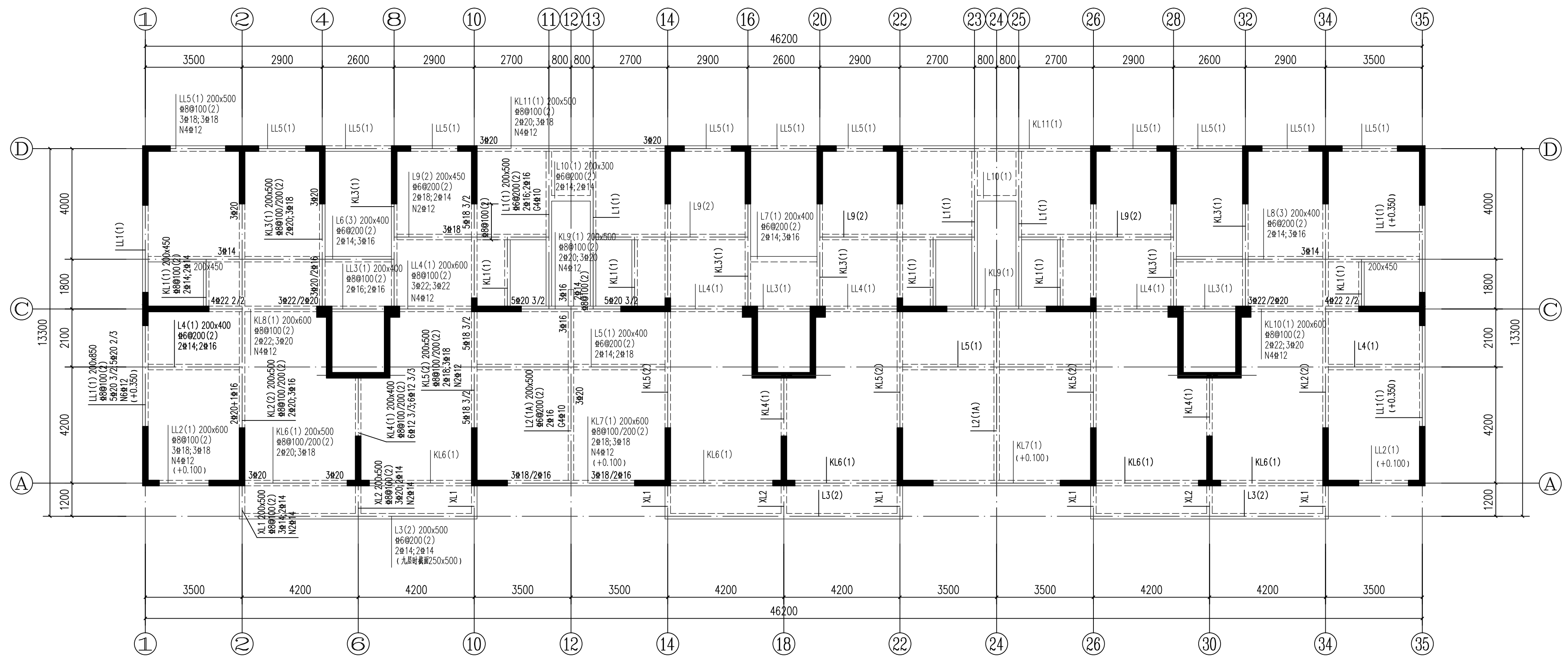
七~九层梁平面图 1:100
